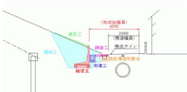
道路拡幅工事 断面図
